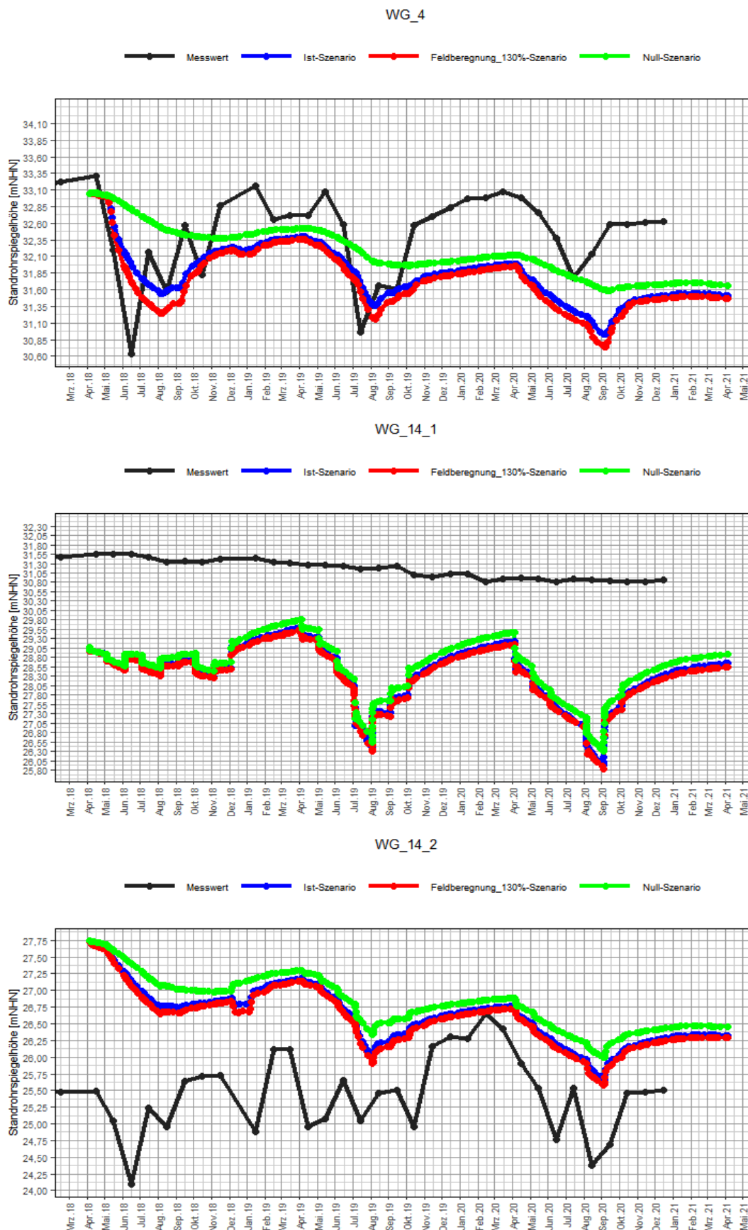
Anlage 4: Vergleich von messwertbasierten und im Rahmen der Modellszenarien simulierten Ganglinien der Standrohrspiegelhöhen für die Grundwassermessstellen in den vier Pilot-Gebieten
